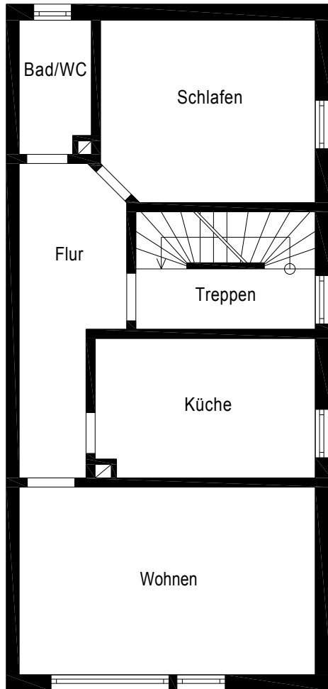
1.Obergeschoss
