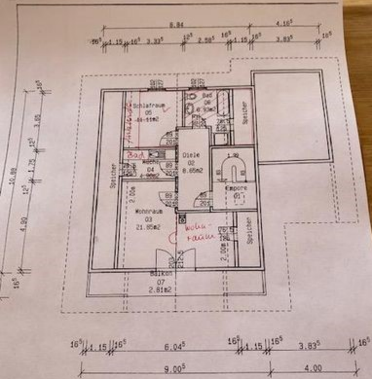
OBERGESCHOSS
