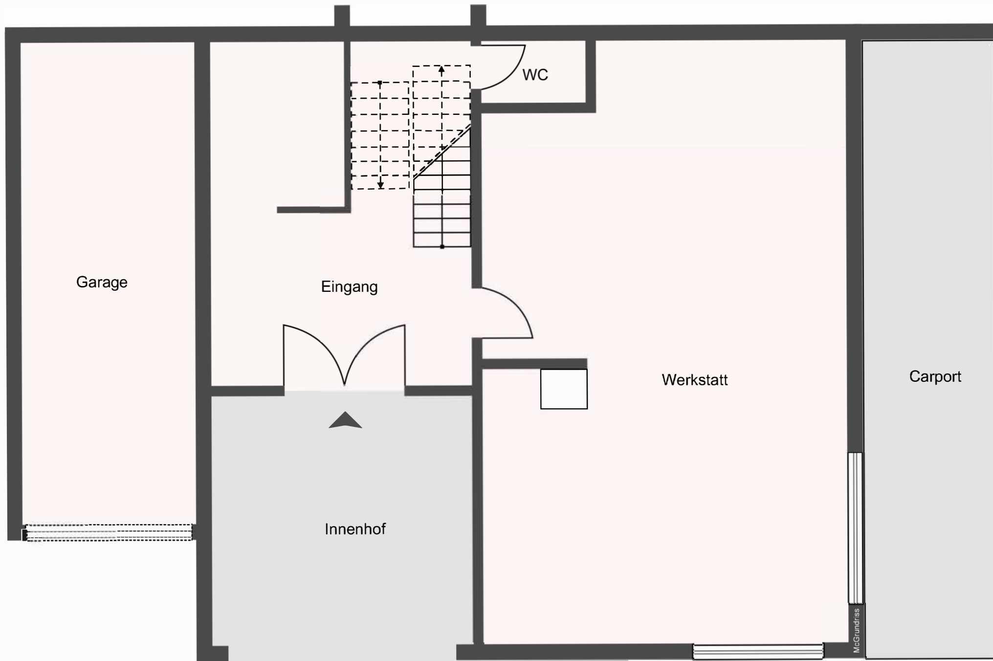
Grundriss Erdgeschoss
